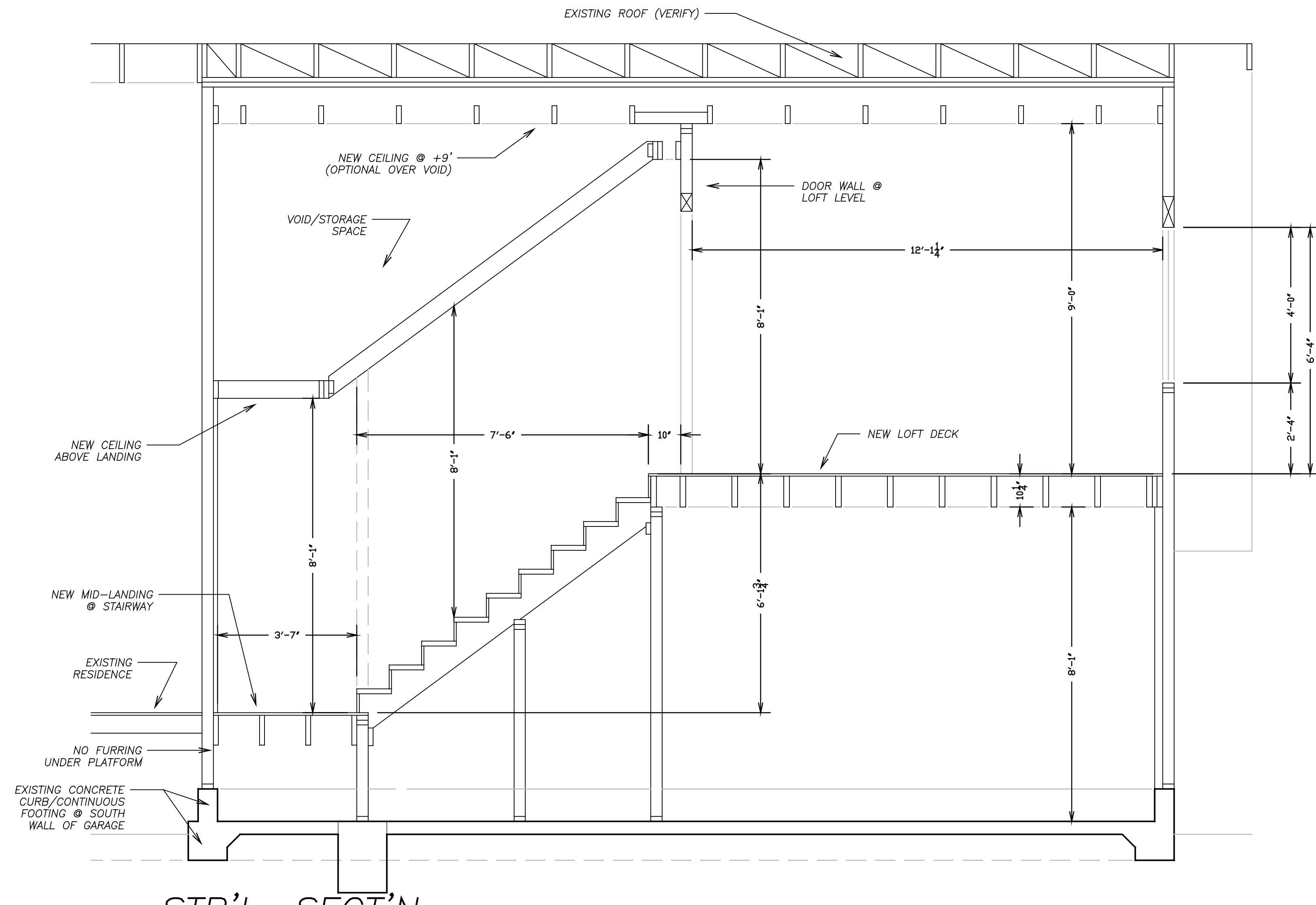
STR'L. SECT'N. @ LANDING/STAIR ① SCALE: 1/2" = 1'-0"
