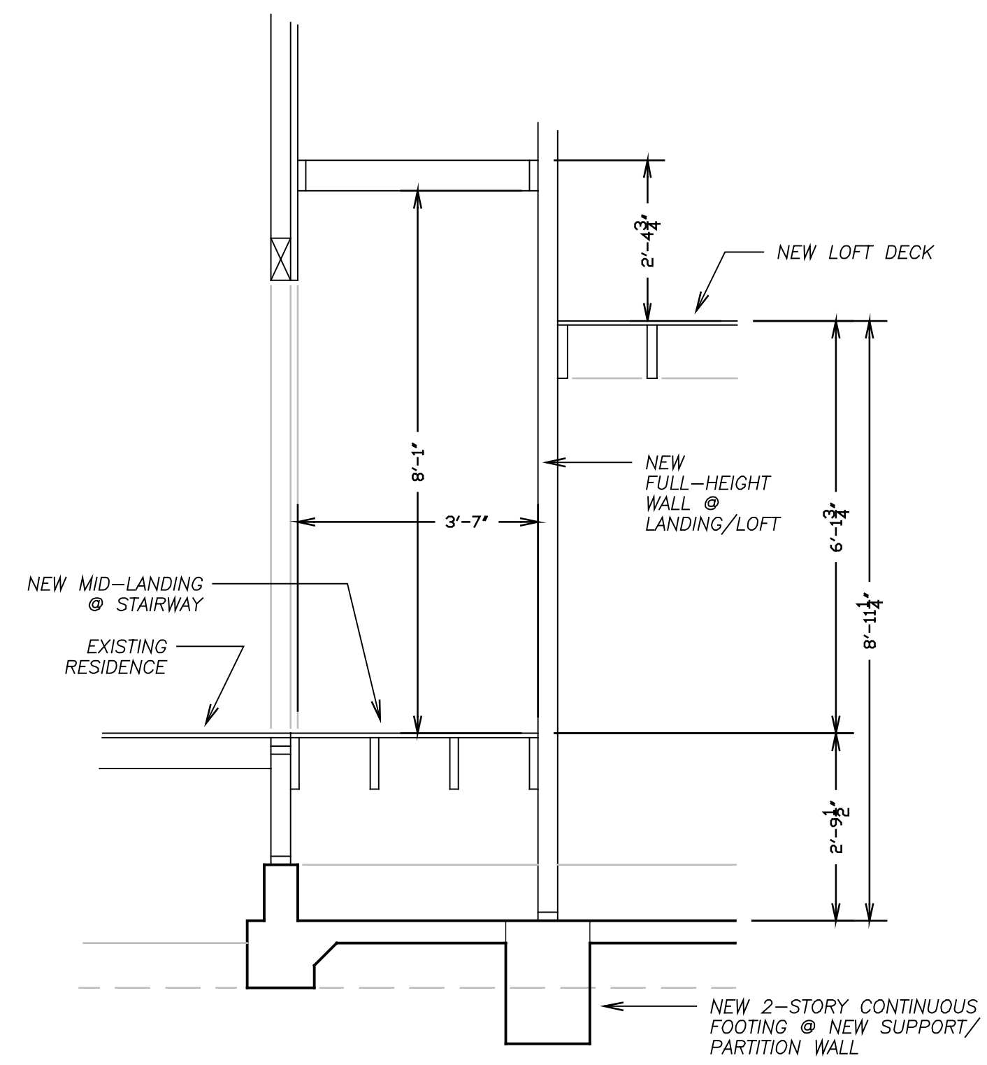
STR'L. SECT'N. @ LANDING/WALL ② SCALE: 1/2" = 1'-0"
